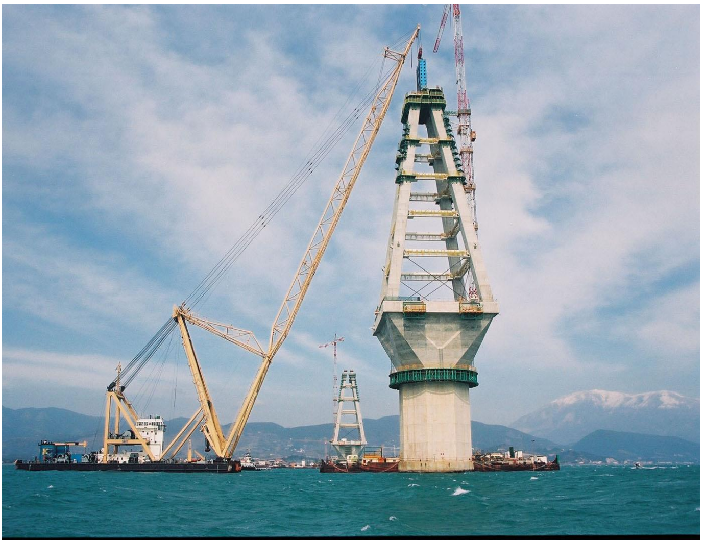
Pose du premier élément de la tête de pylône
