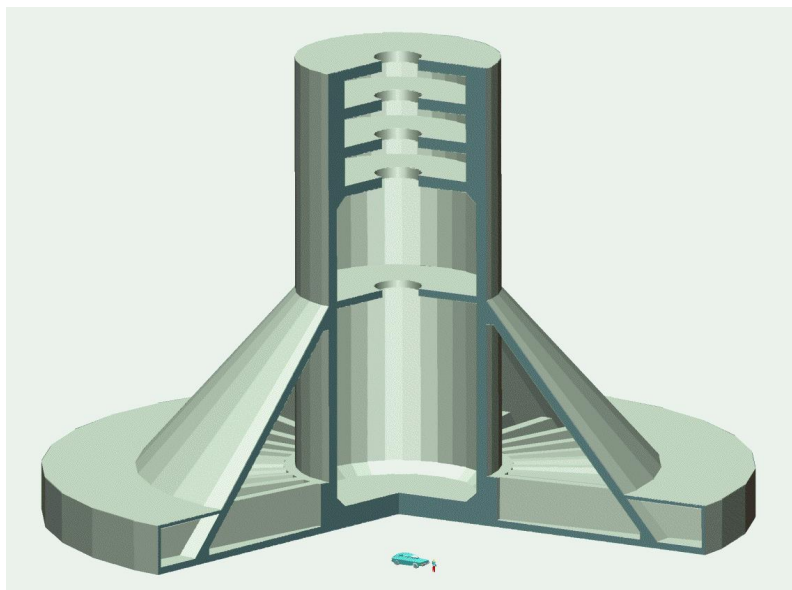
Vue d'un caisson de fondation, une voiture pour donner l'échelle
