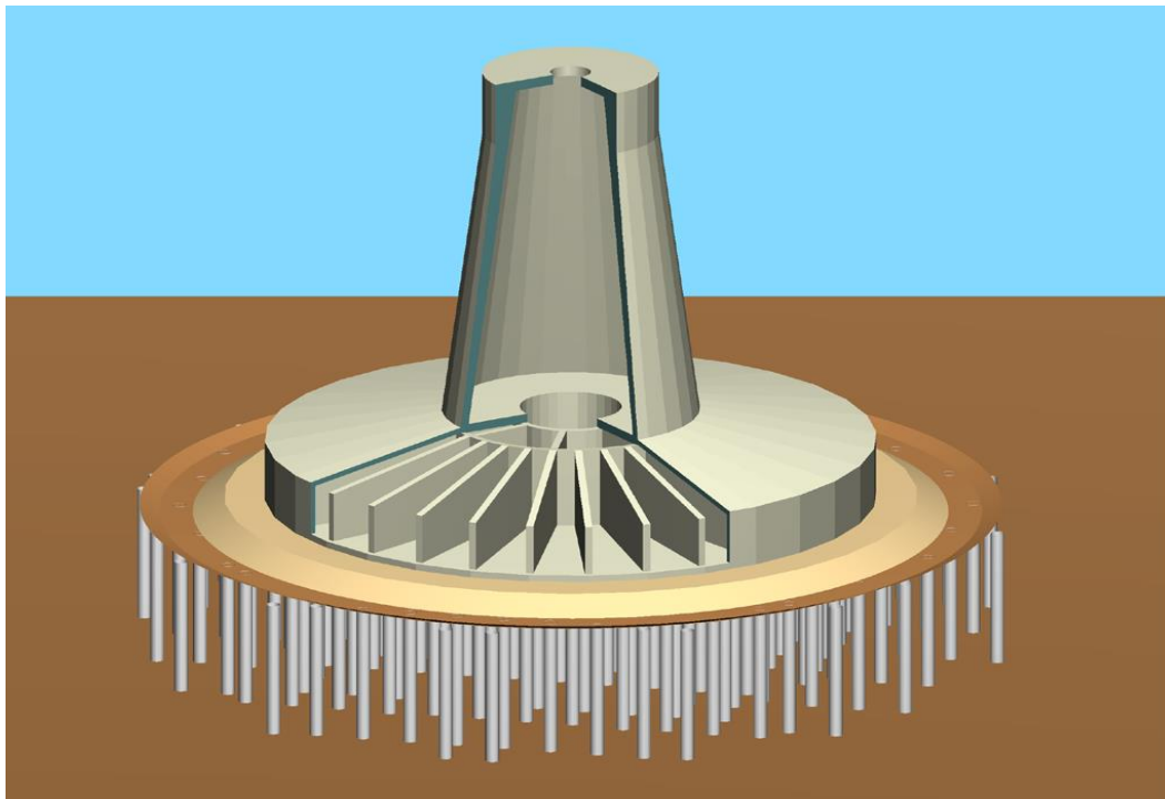
Vue des nouveaux caissons de fondation, avec les inclusions
